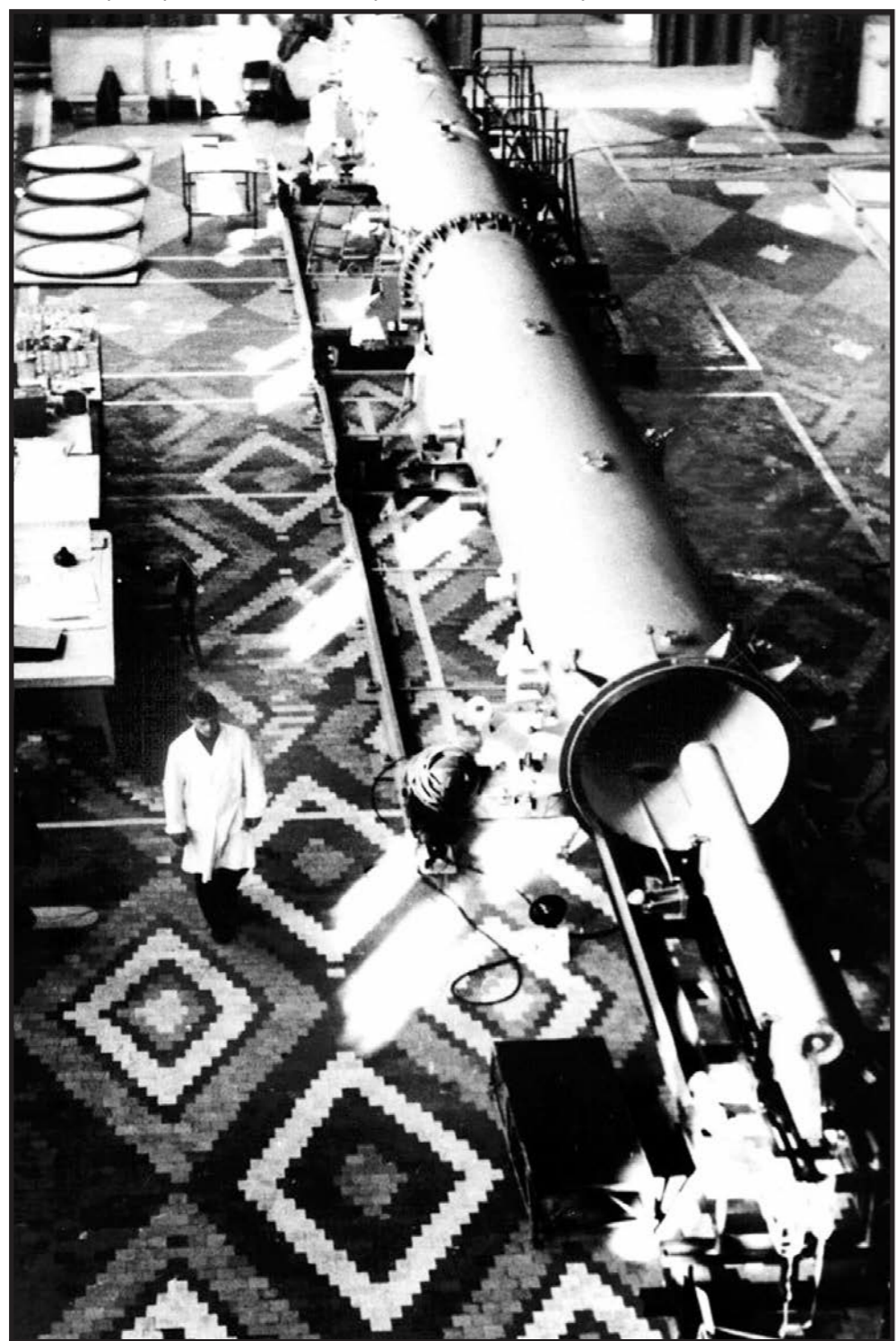
Взрывной фотодиссоционный лазер Ф-1200 проекта ВНИИЭФ
