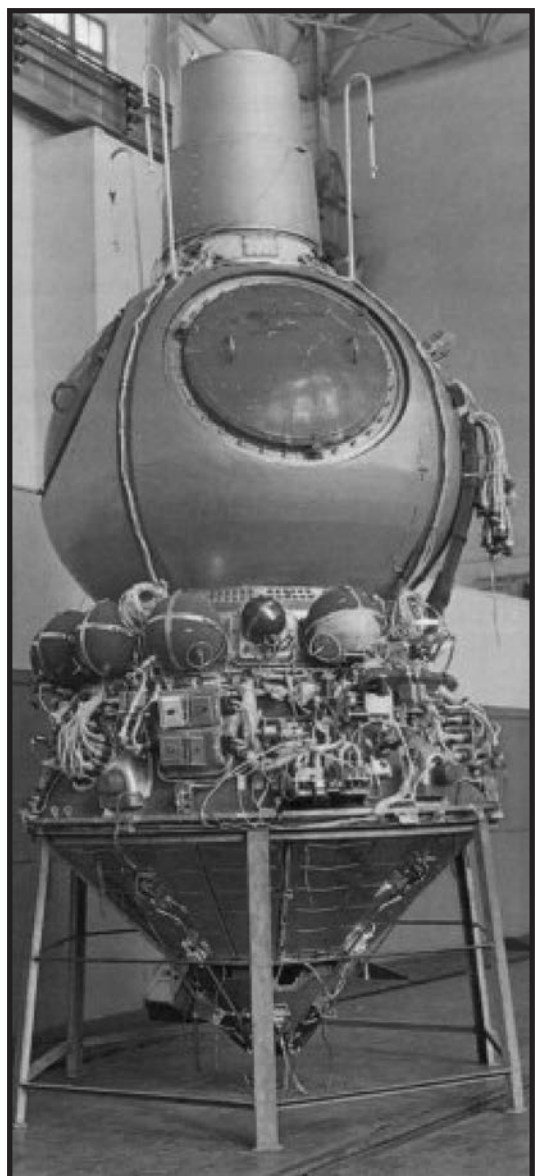
Многоместный космический корабль «Восход» (ЗКВ); 1964 год. РКК «Энергия»
