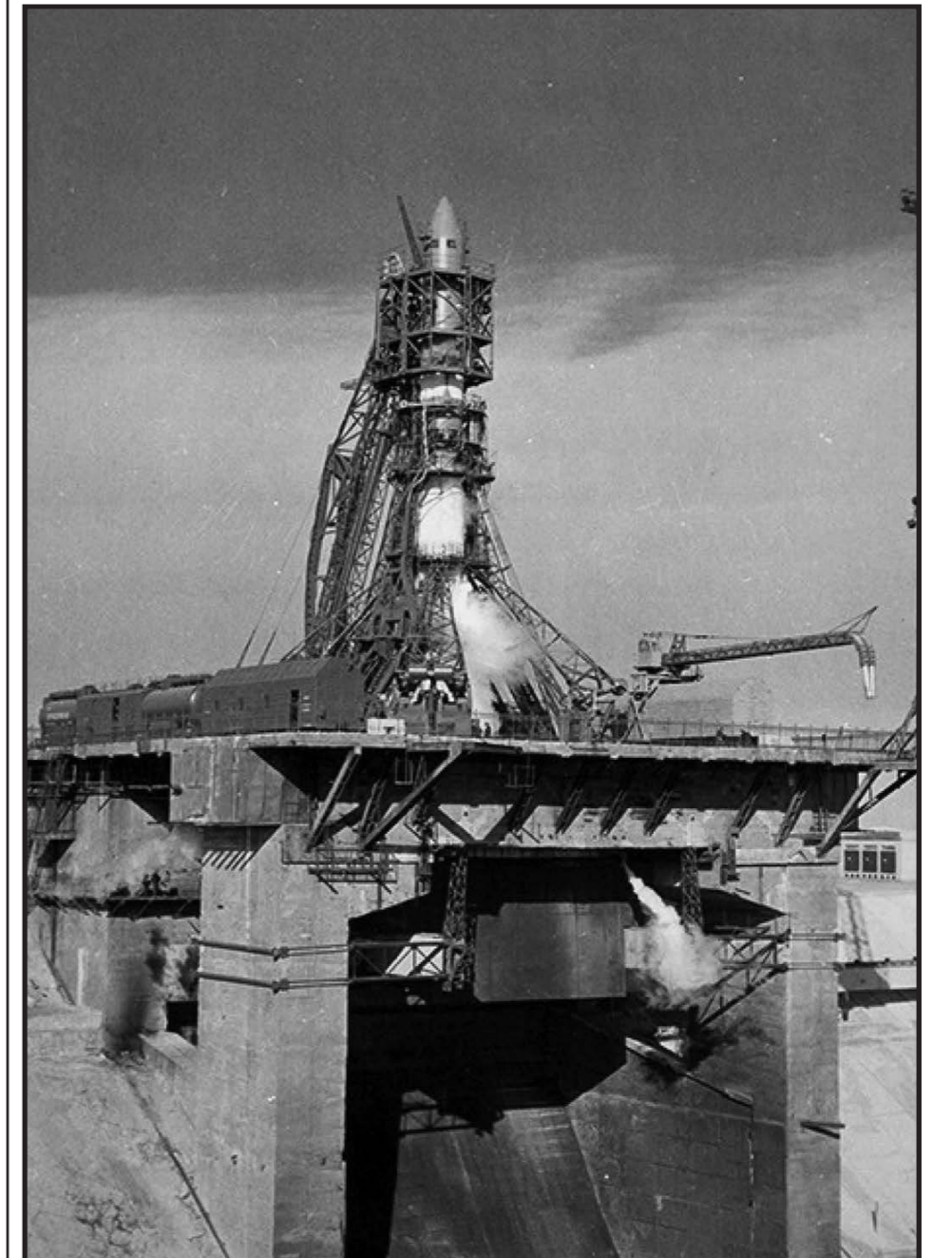
Ракета-носитель «Восход» (11А57) с космическим кораблём «Восход» (ЗКВ №3) на стартовом комплексе; 12 октября 1964 года
